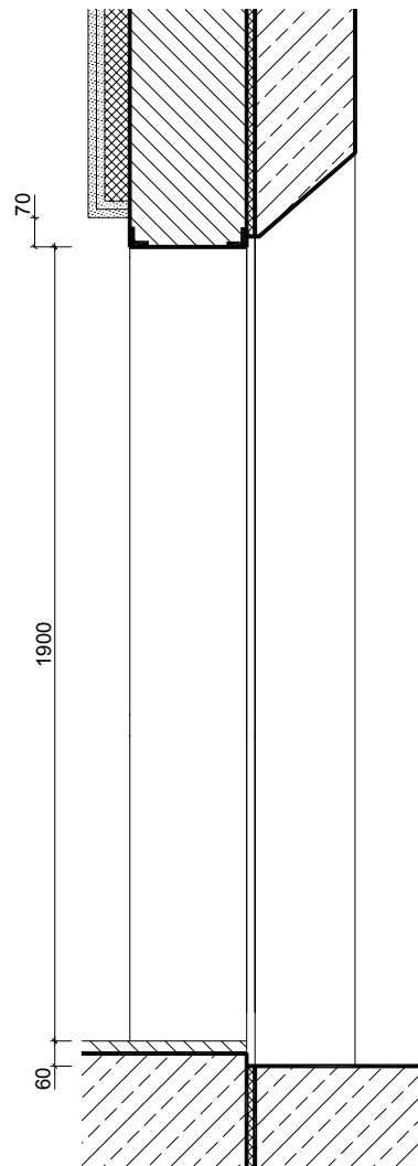
VERTIKALSCHNITT
