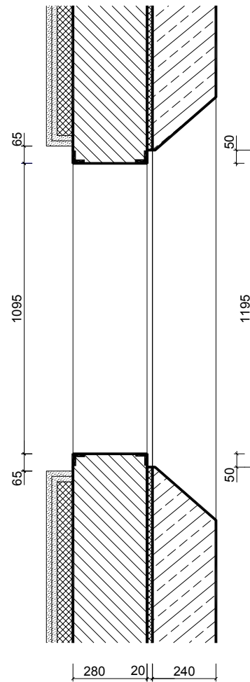
HORIZONTALSCHNITT
